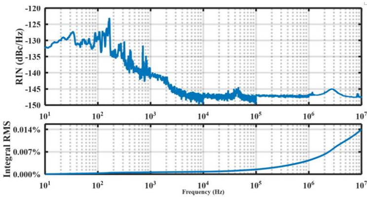
相对强度噪声测试 (RIN) : 0.014% [10Hz-10MHz]
