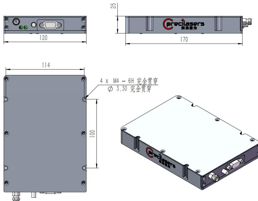
产品尺寸图-小体积版本
