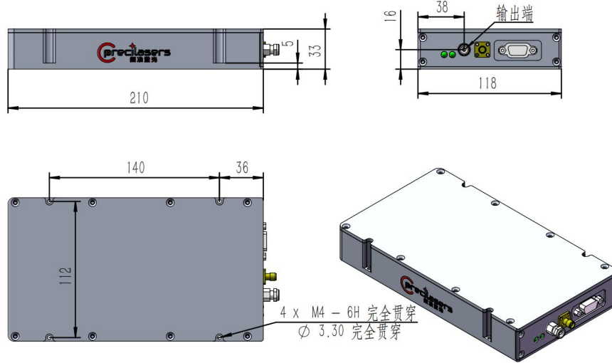
产品尺寸图-常规
