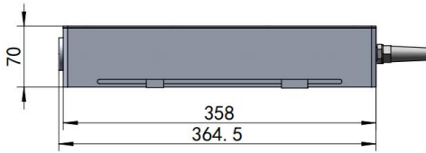
激光头尺寸
