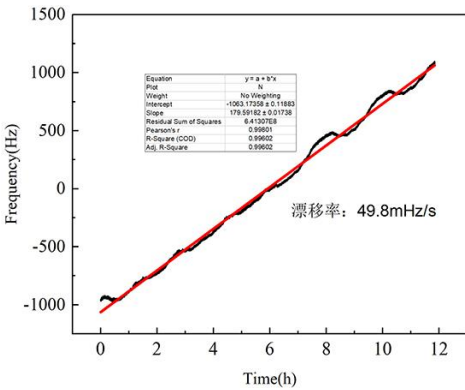
频率漂移测试
