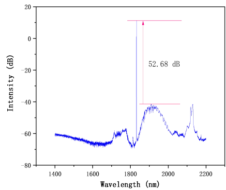
光谱测试图
