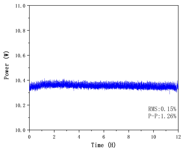
功率稳定测试图
