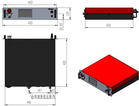
机箱尺寸图-水冷
