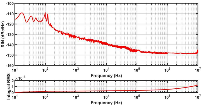
RIN噪声测试图
